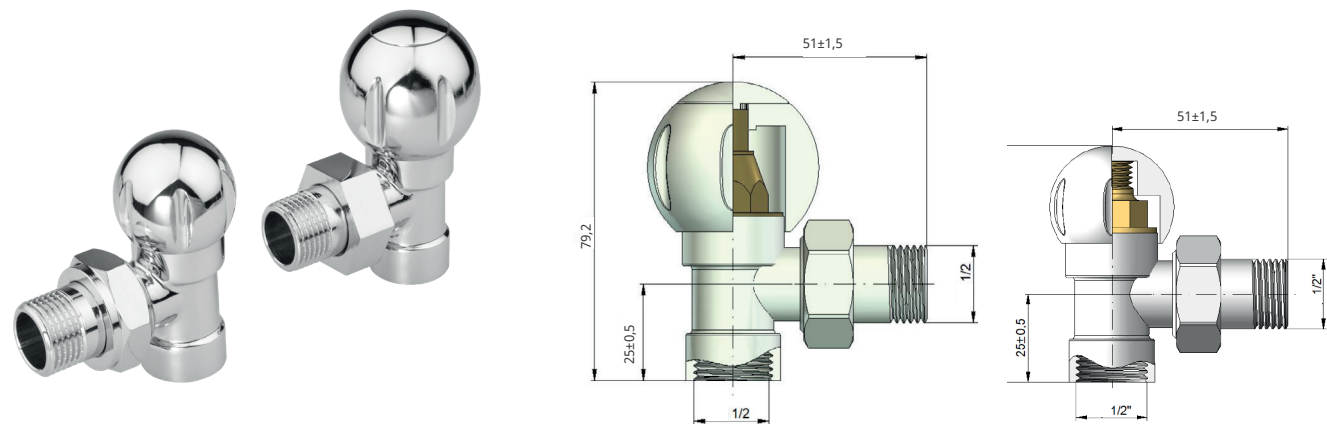
Регулювальний (ручний) комплект BALL, кутовий, ВР 1/2" / ЗР 1/2". Склад комплекту: регулювальний (ручний) кран BALL, зворотній клапан BALL.
